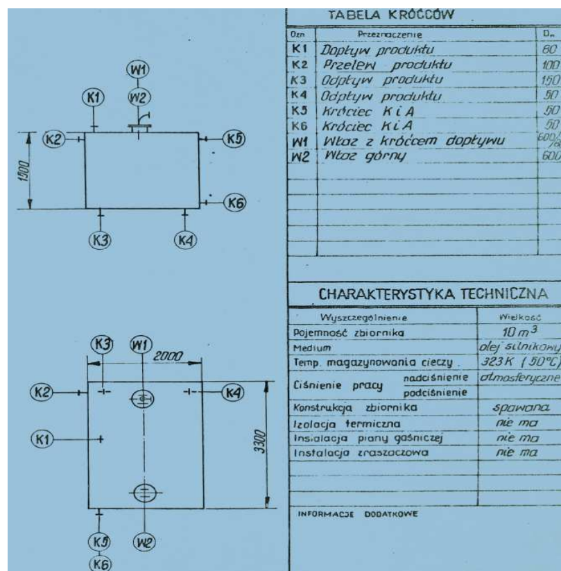
Rysunek 1: Charakterystyka techniczna zbiorników
